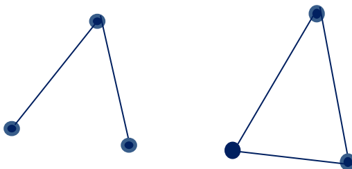
Графы G_1 G_2 , изоморфизм которых требуется установить
